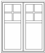
2-Luft SP 1:0 - 55 + SP 1:1
